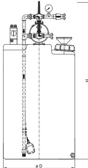
Abmessungen Küwamat R -X -MBE
